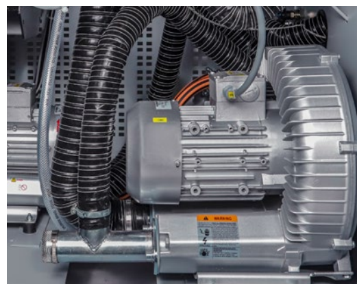
Turbine à canal latéral
