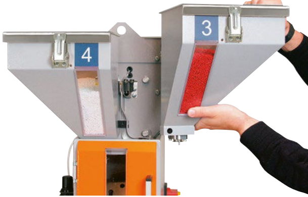
GRAVICOLOR 30 MD, sökülebilir besleme haznesi
